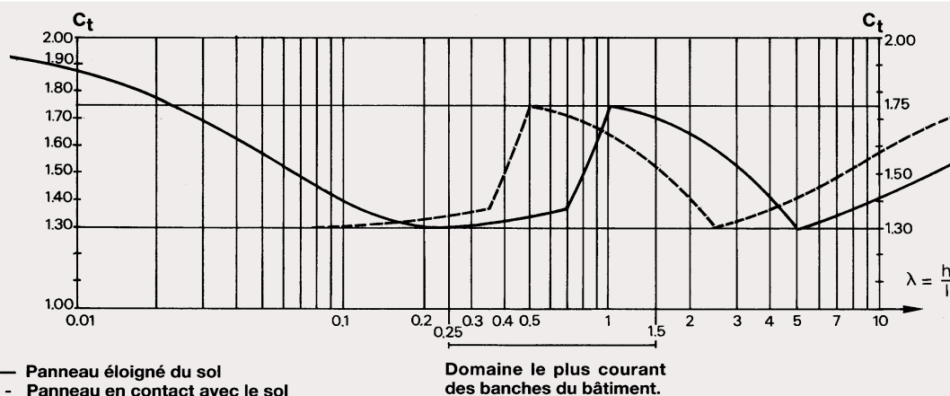
Fig. 3 Valeurs du coefficient de traînée fournies par les règles Neige et Vent. Panneaux pleins, lisses, rectangulaires, en contact ou non avec le sol.
